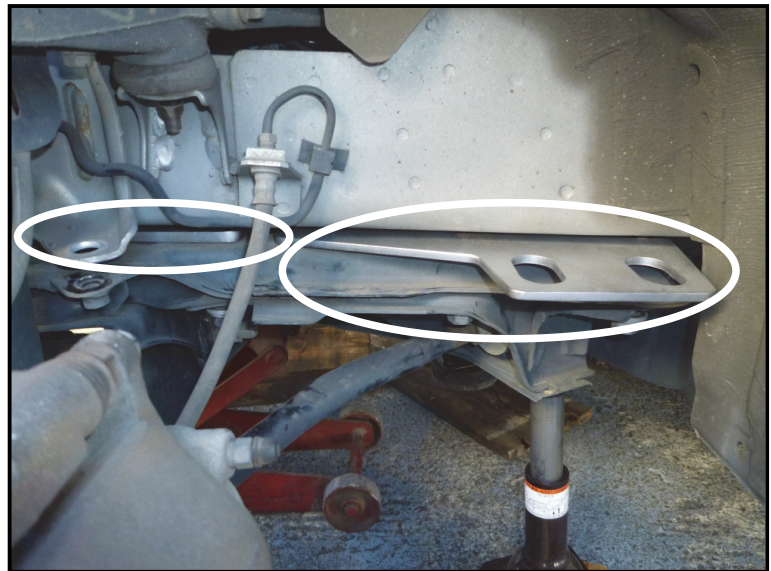
左にスペーサー、右に固定ジグ本体(車両左側の場合)
