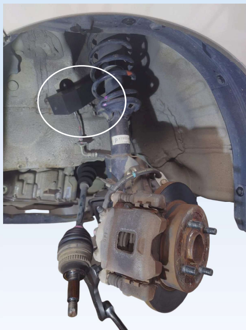
【ショックを保持している例】
