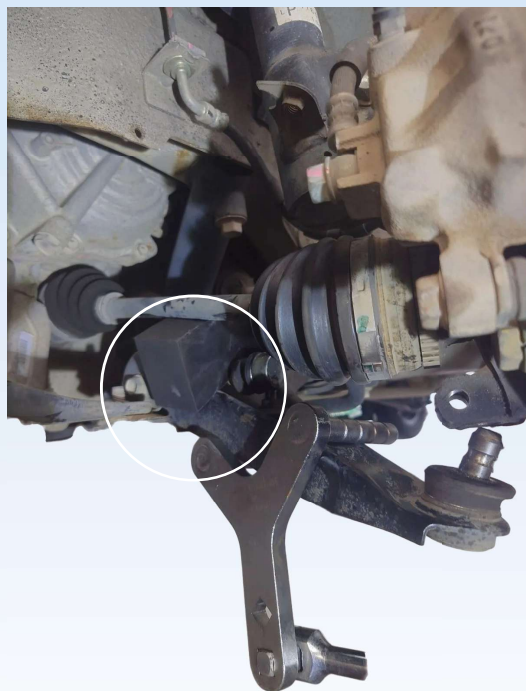
【ロアアームを保持している例】
