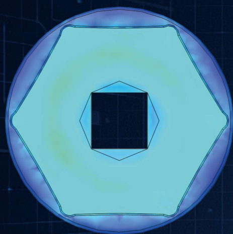
応力解析結果
