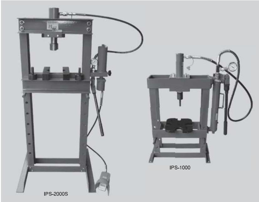
ケース外形寸法 ●IPS-1000 W755×L550×H185 / 55kg ●IPS-1000S W1740×L520×H320 / 170kg ●IPS-2000S W1740×L520×H320 / 181kg
